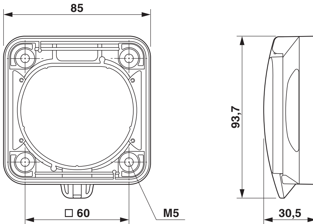
Rysunek wymiarowy
