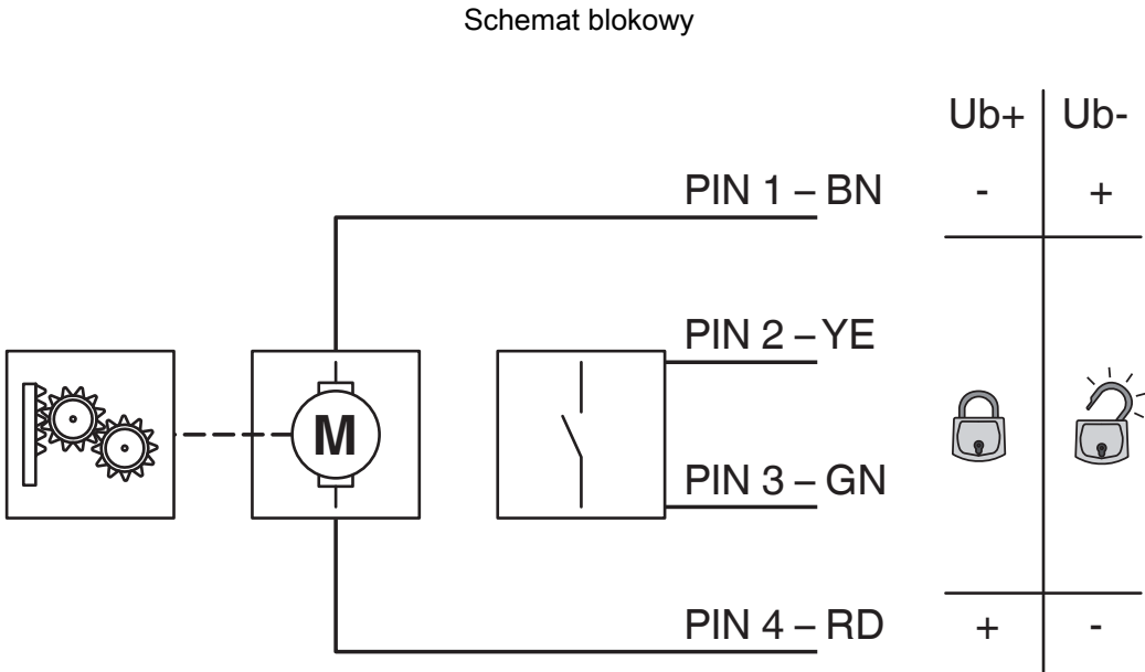
Schemat blokowy siłownika blokady
