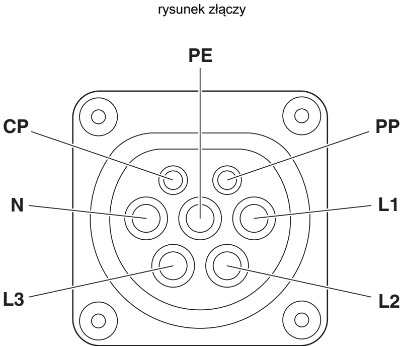
Przyporządkowanie pinów infrastrukturalnego gniazda ładowania
