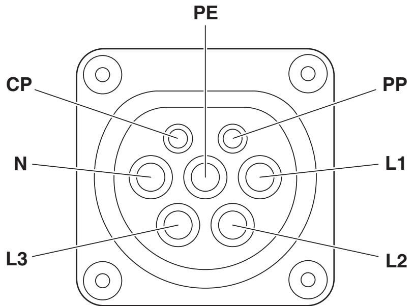
Przyporządkowanie pinów infrastrukturalnego gniazda ładowania
