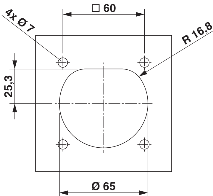
Rysunek wymiarowy
