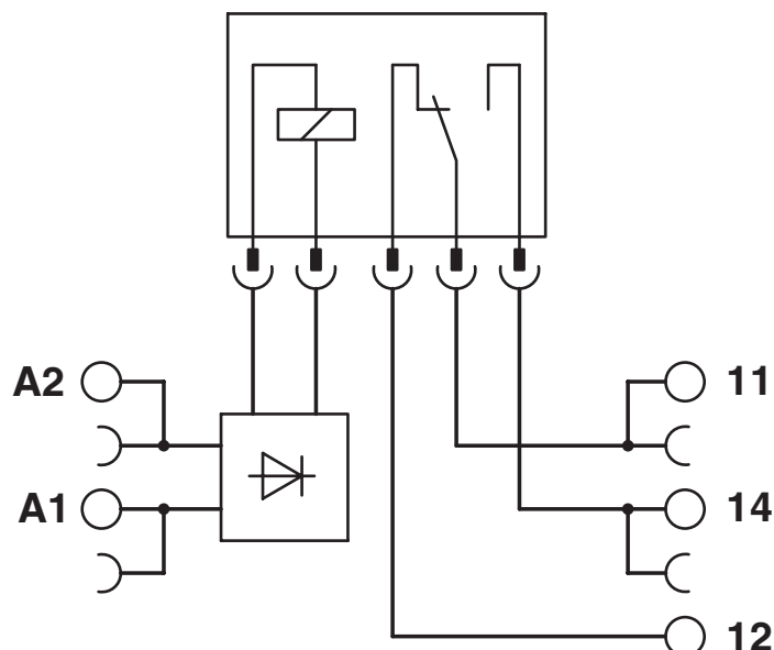
Schemat
