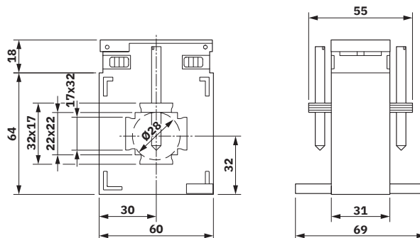
Rysunek wymiarowy
