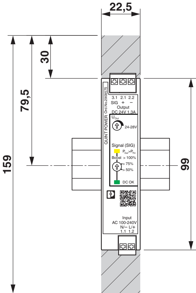
Rysunek wymiarowy
