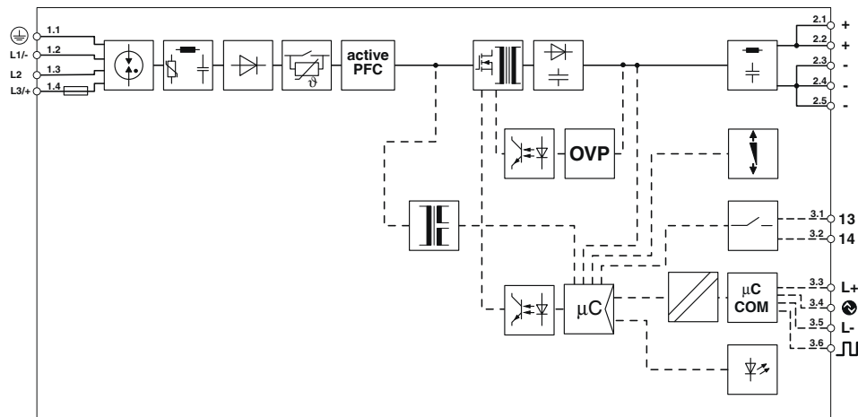
Schemat blokowy
