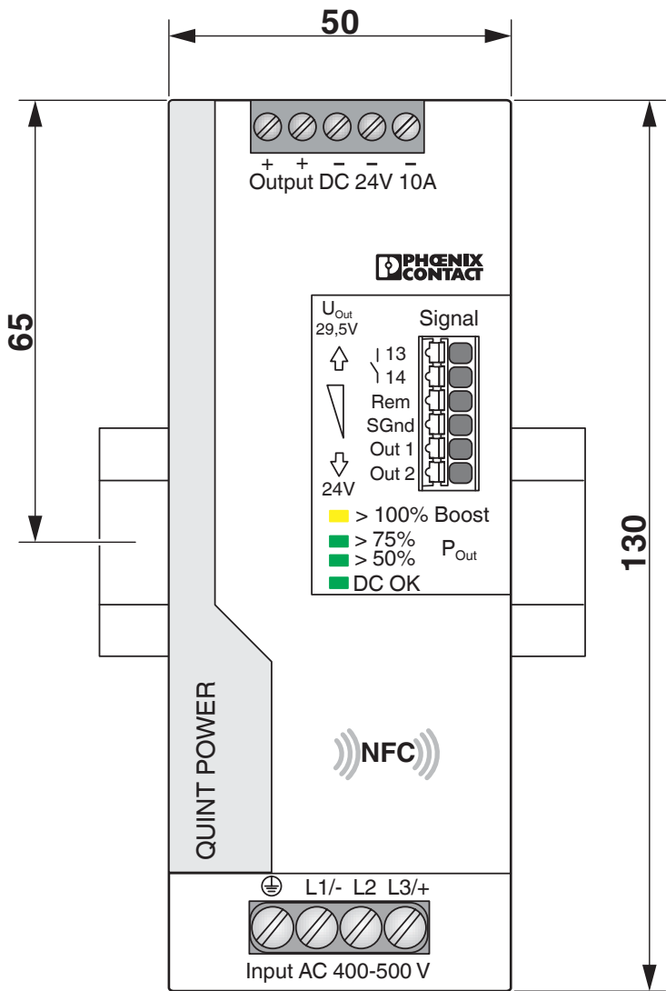
Rysunek wymiarowy
