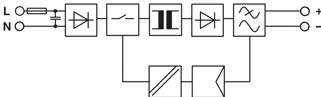
Schemat blokowy
