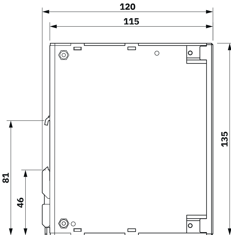
Rysunek wymiarowy
