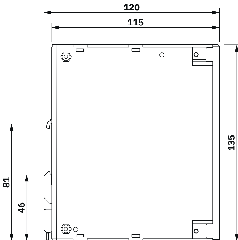
Rysunek wymiarowy
