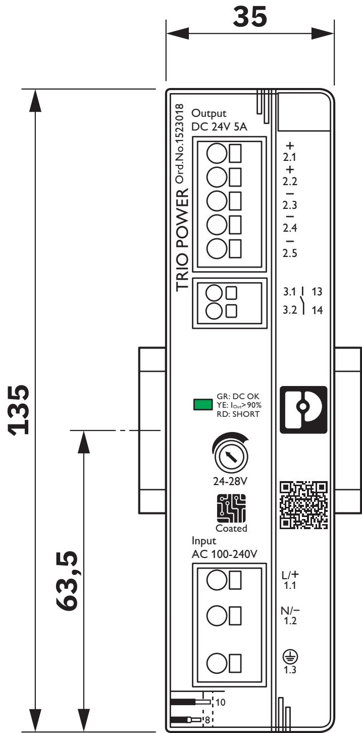
Rysunek wymiarowy
