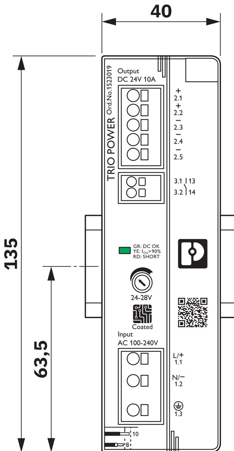
Rysunek wymiarowy
