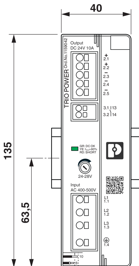
Rysunek wymiarowy
