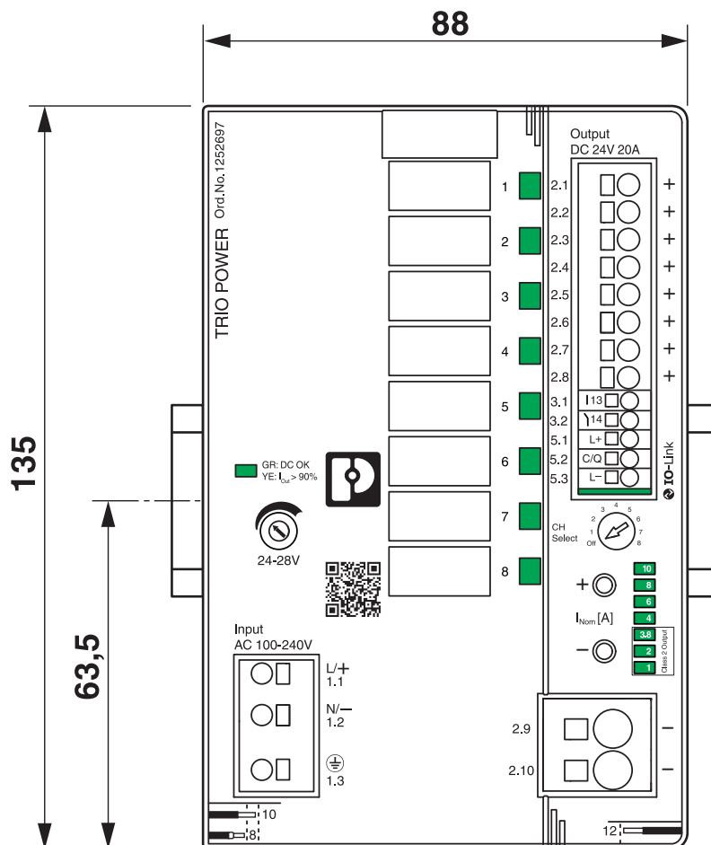
Rysunek wymiarowy
