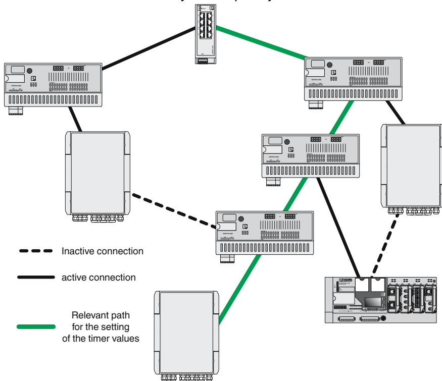
rysunek aplikacji
