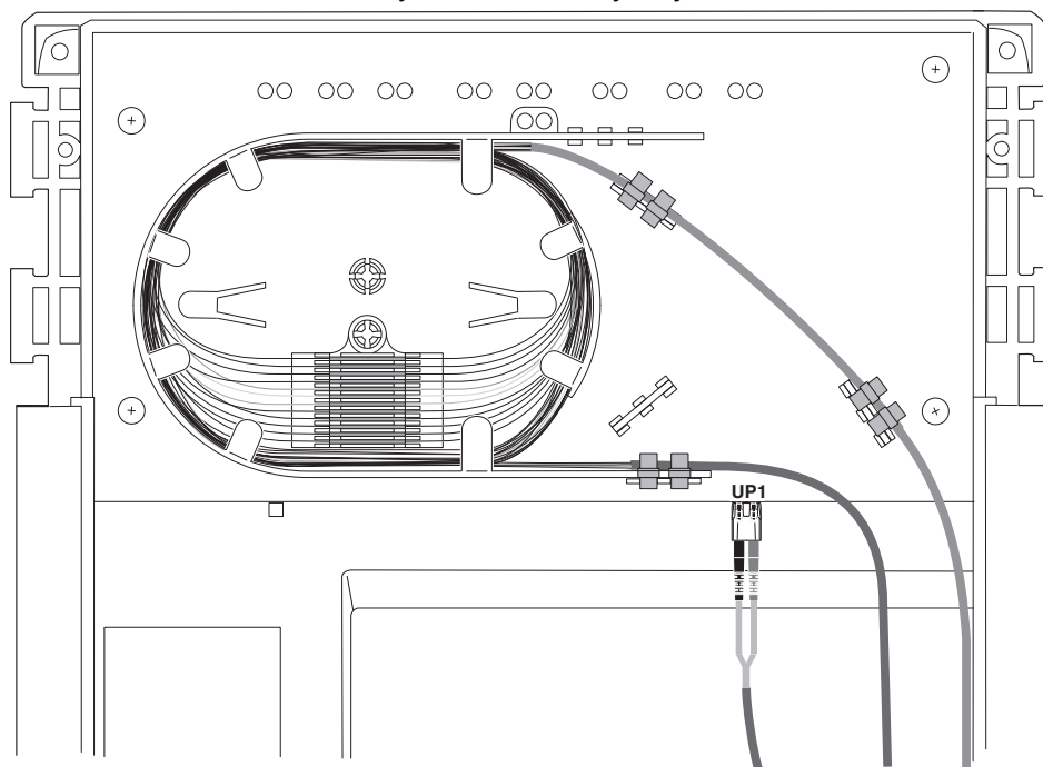
Rysunek schematyczny
