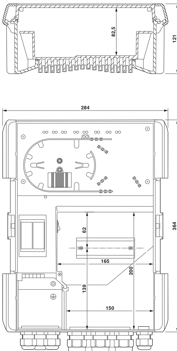
Rysunek wymiarowy
